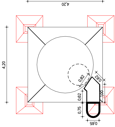
Planta Baixa c/ reservatório esc. 1:100
