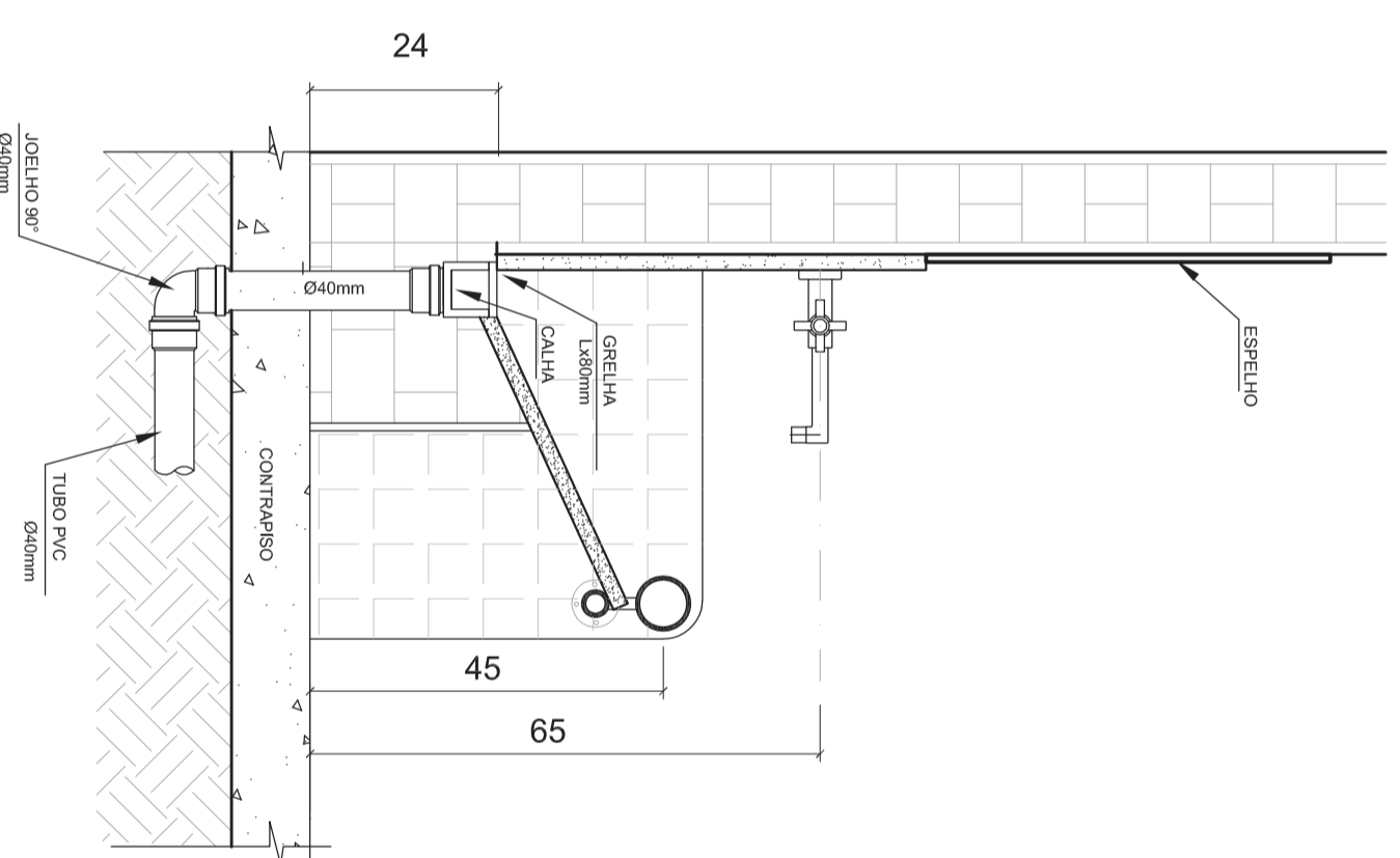
DETALHE TUBULAÇÃO PIA INFANTIL CORTE TRANSVERSAL ESCALA: 1/10
