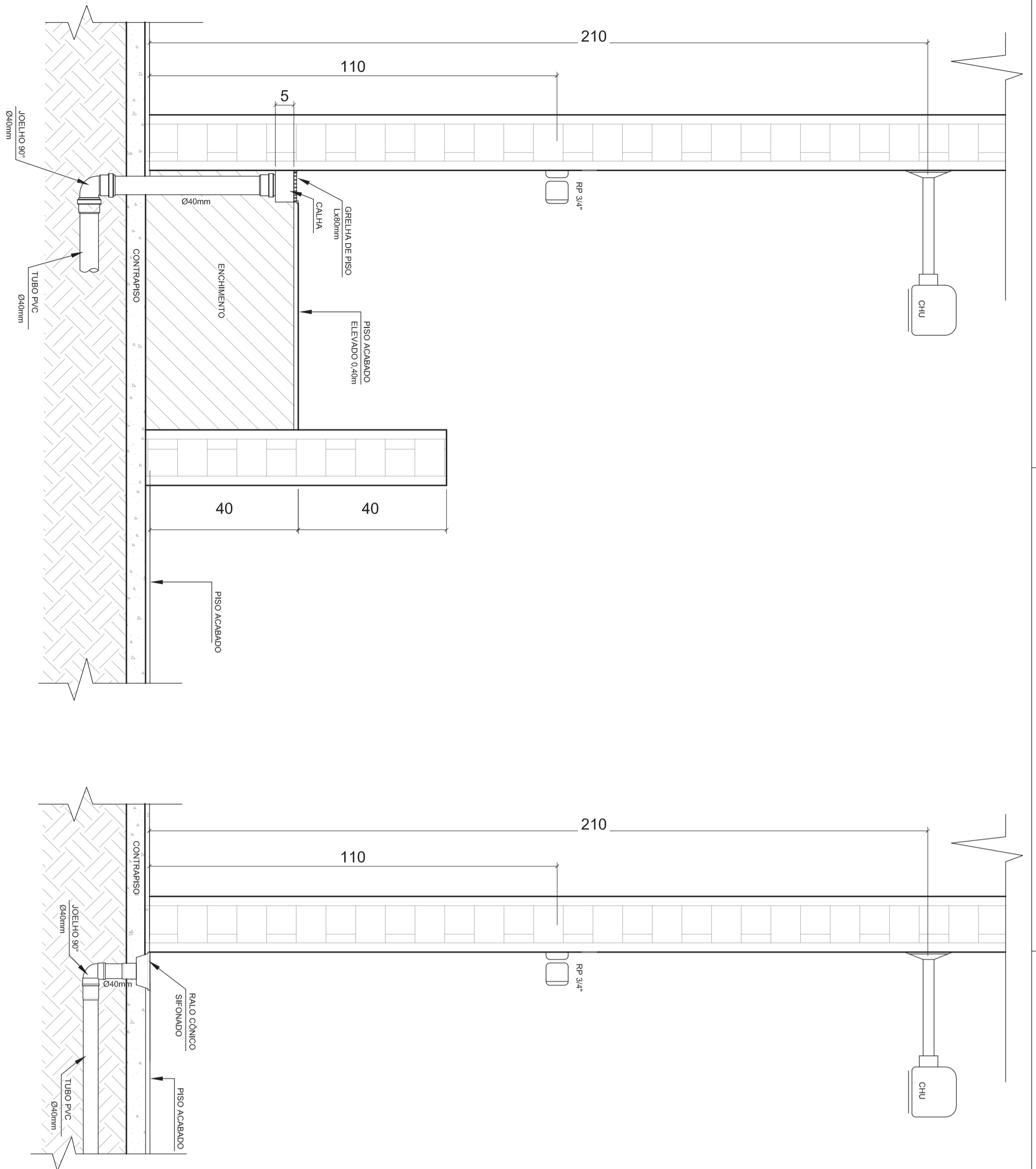
DETALHE DOS CHUVEIROS INFANTIS - RAMAL DE ESGOTO CORTE TRANSVERSAL ESCALA: 1/10
