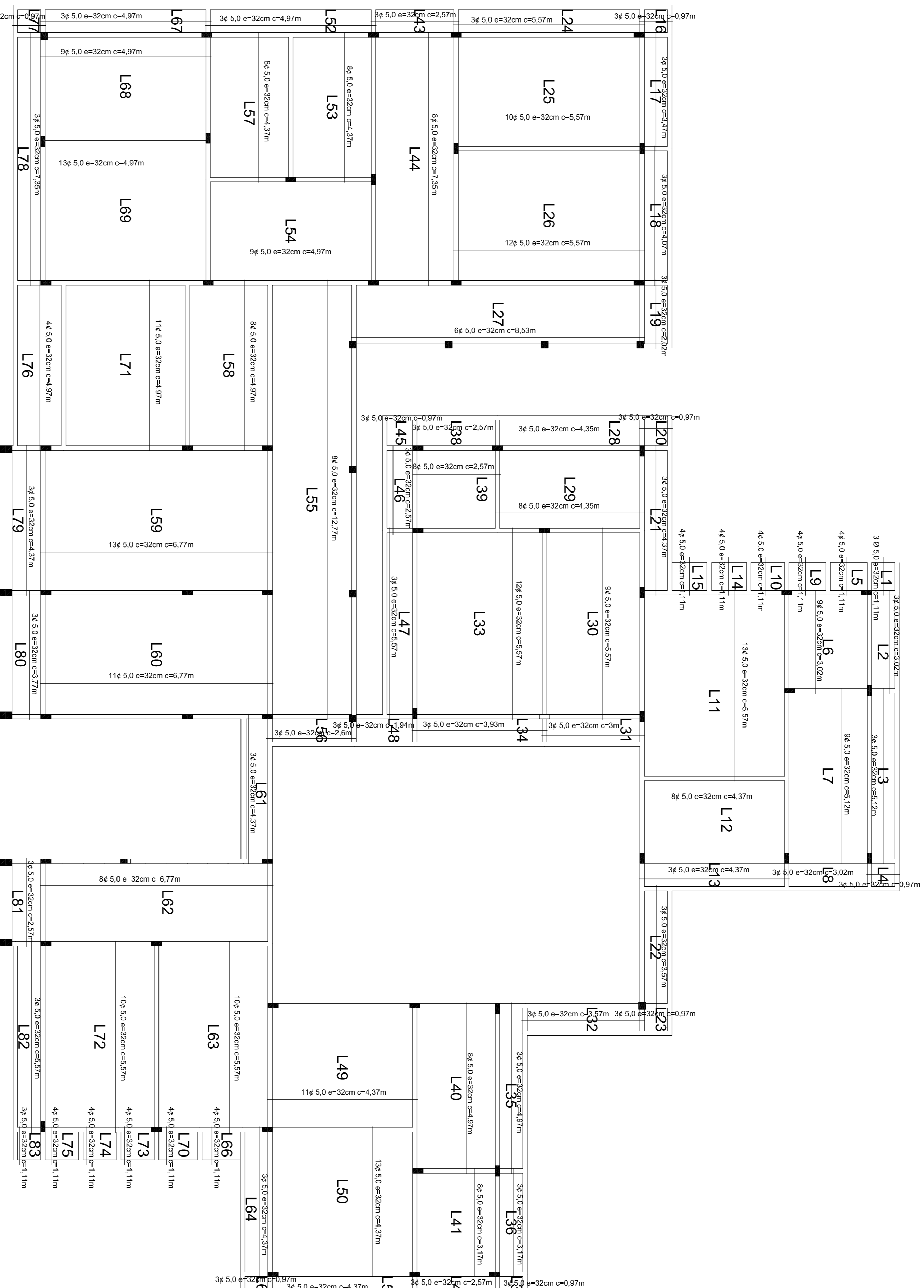
ARMADILHA DE DISTRIBUIÇÃO - LAJES DA COBERTURA ESCALA: 1/75
