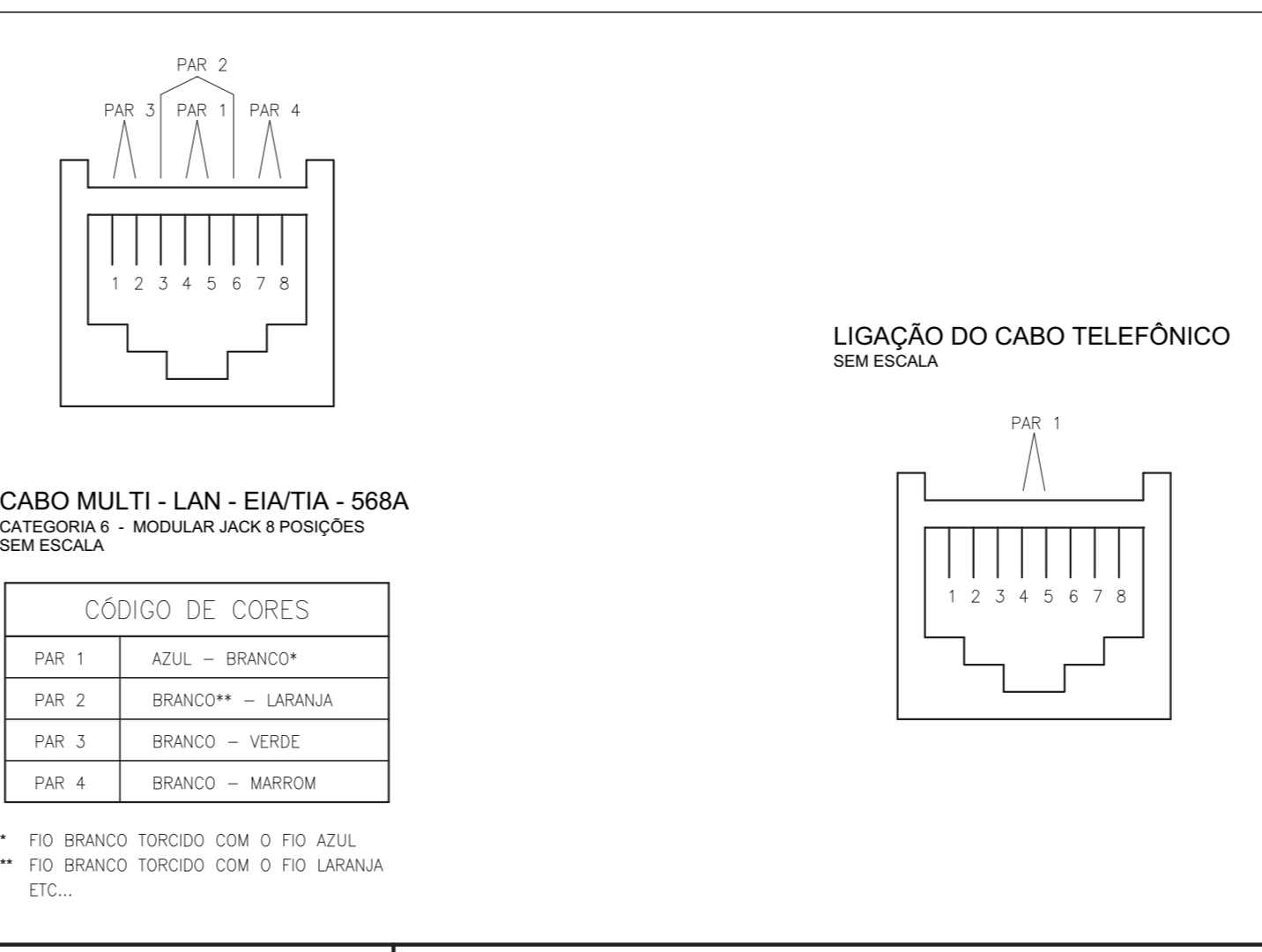
EXEMPLO DE LIGAÇÃO LÓGICA SEM ESCALA
