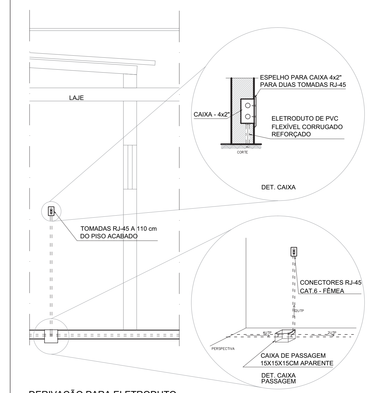
DERIVAÇÃO PARA ELETRODUTO DETALHE GÊNÉRICO
