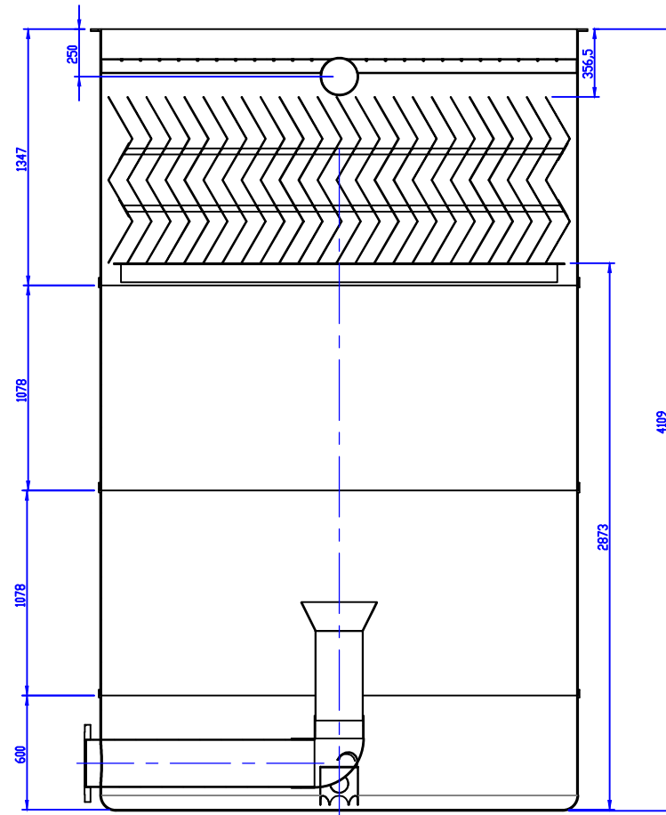
SEÇÃO A-A
