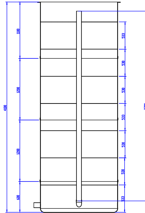
SEÇÃO A-A
