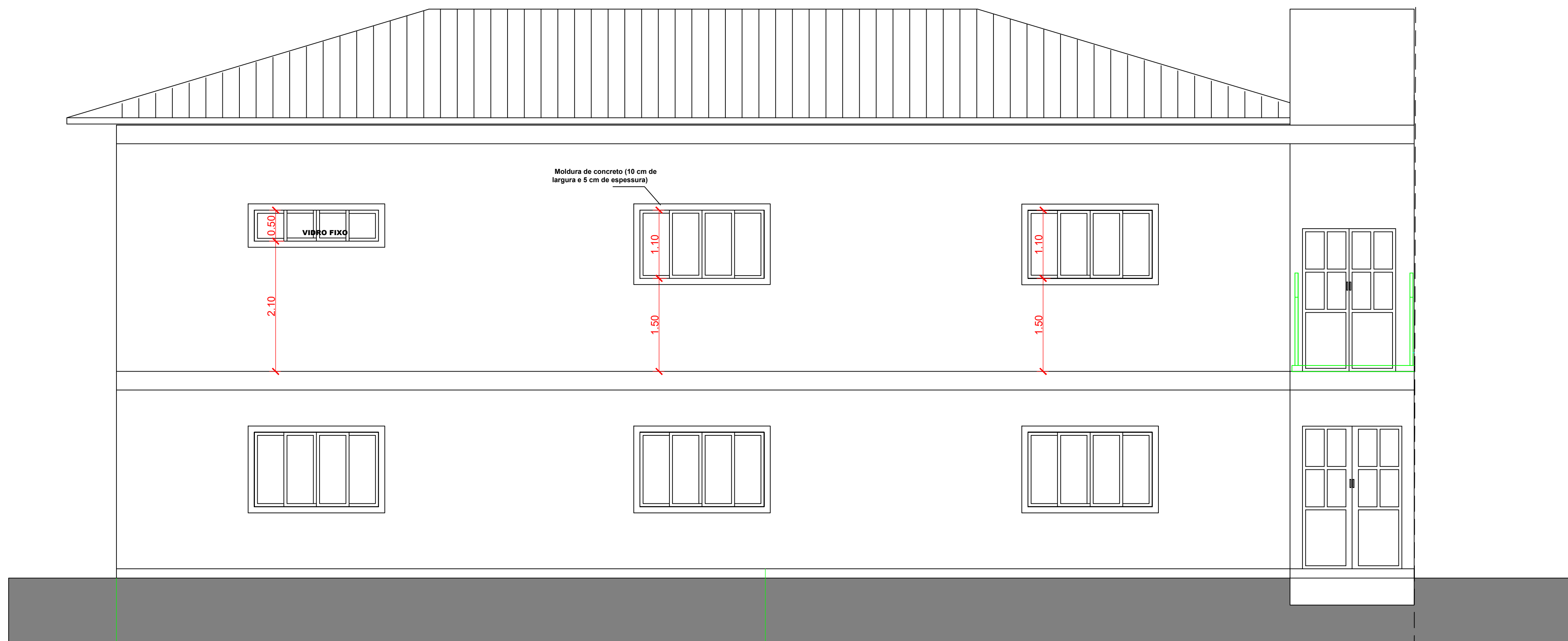
FACHADA PRINCIPAL ESCALA ..... 1:50
