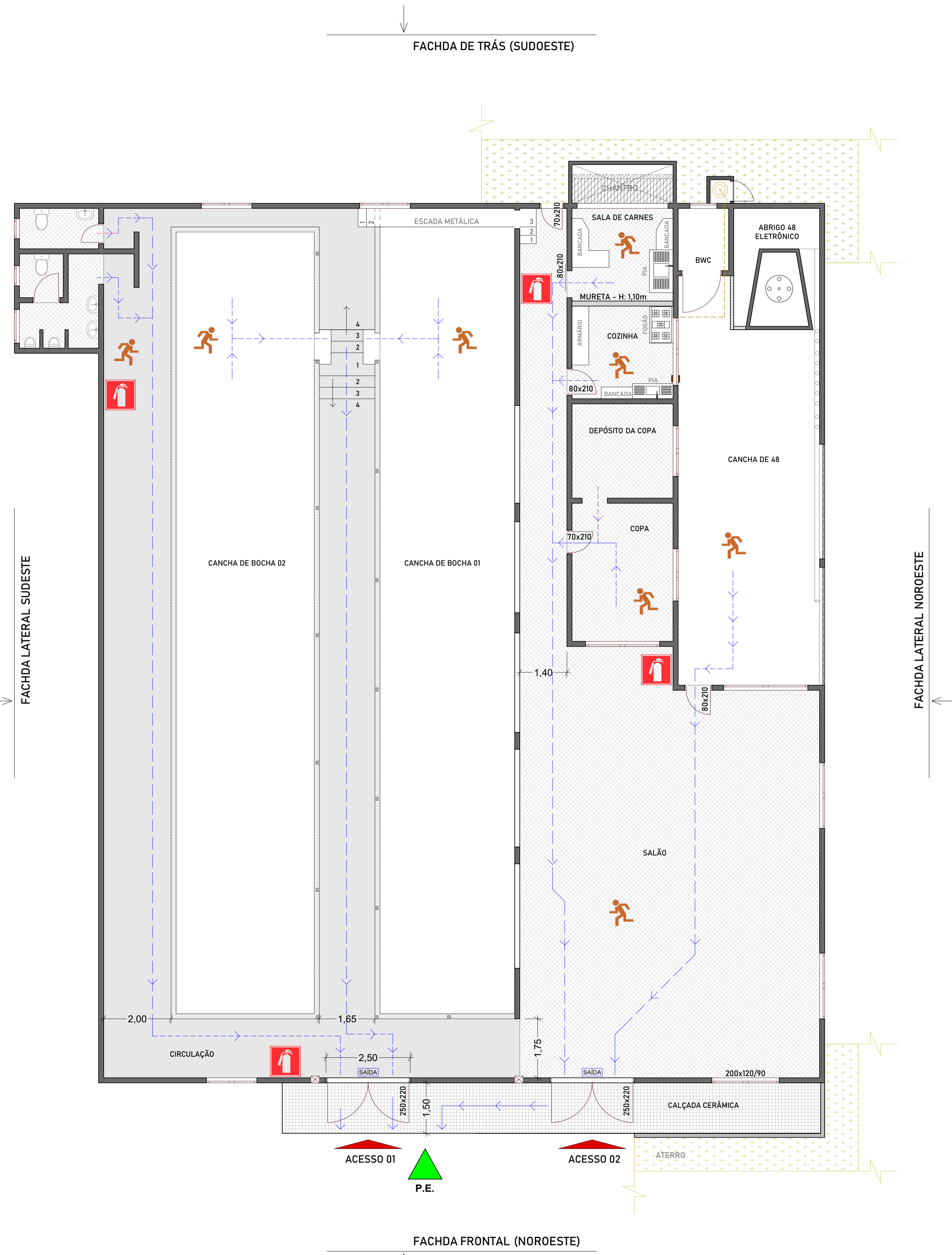
03 PLANTA DE EMERGÊNCIA Escala: 1/75
