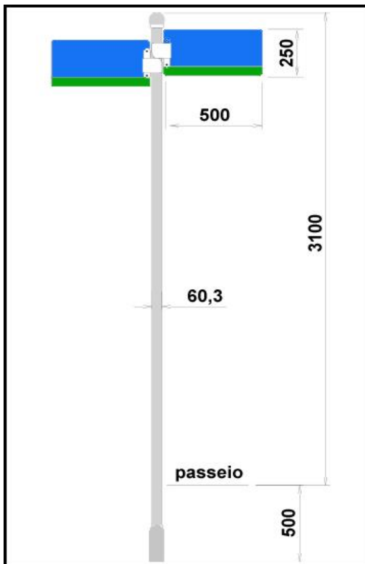
Ilustração 2: Detalhe do poste (medidas em mm)
