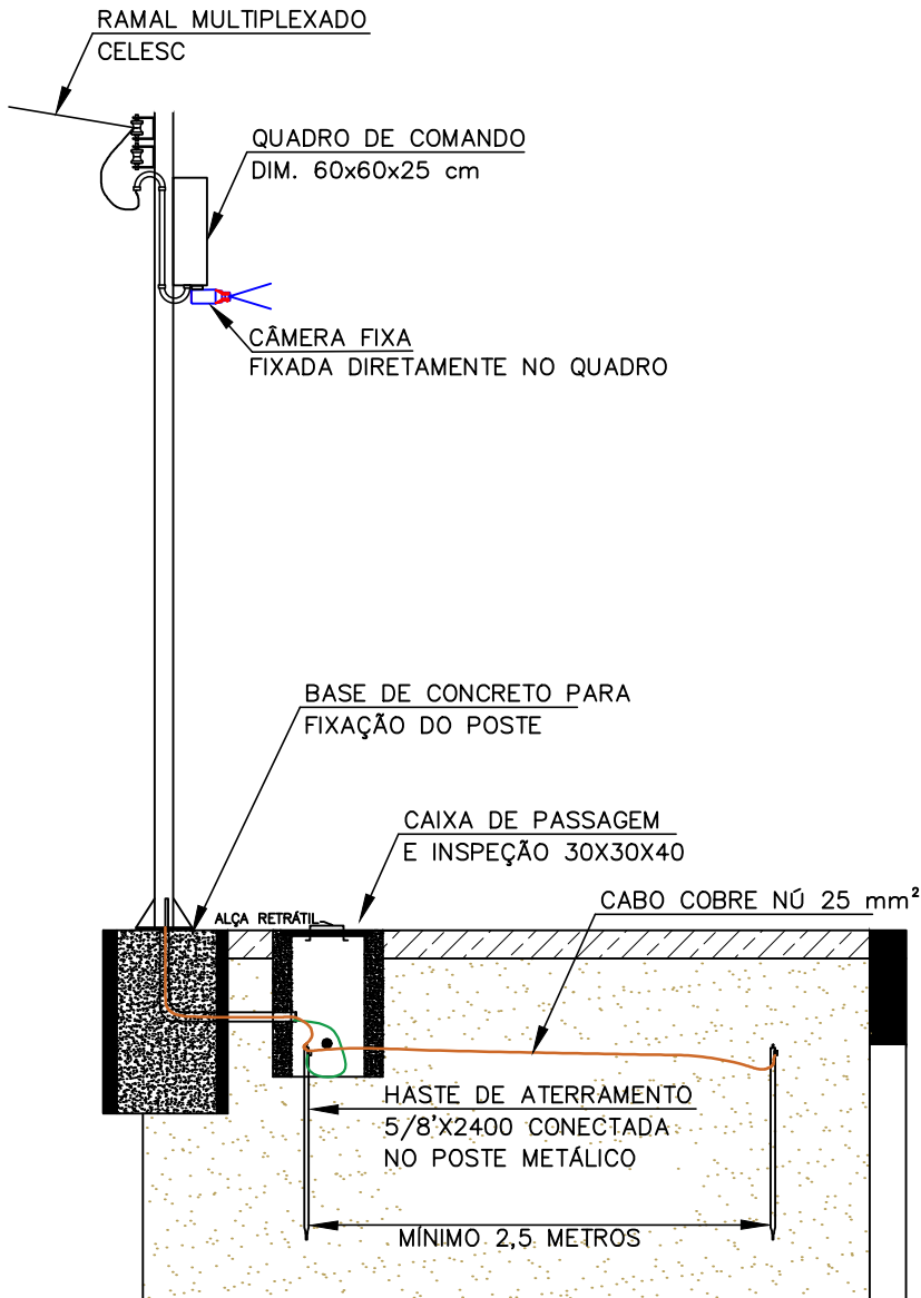
DETALHES INSTALAÇÃO POSTE SEM ESCALA
