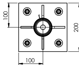
DETALHES FLANGE
