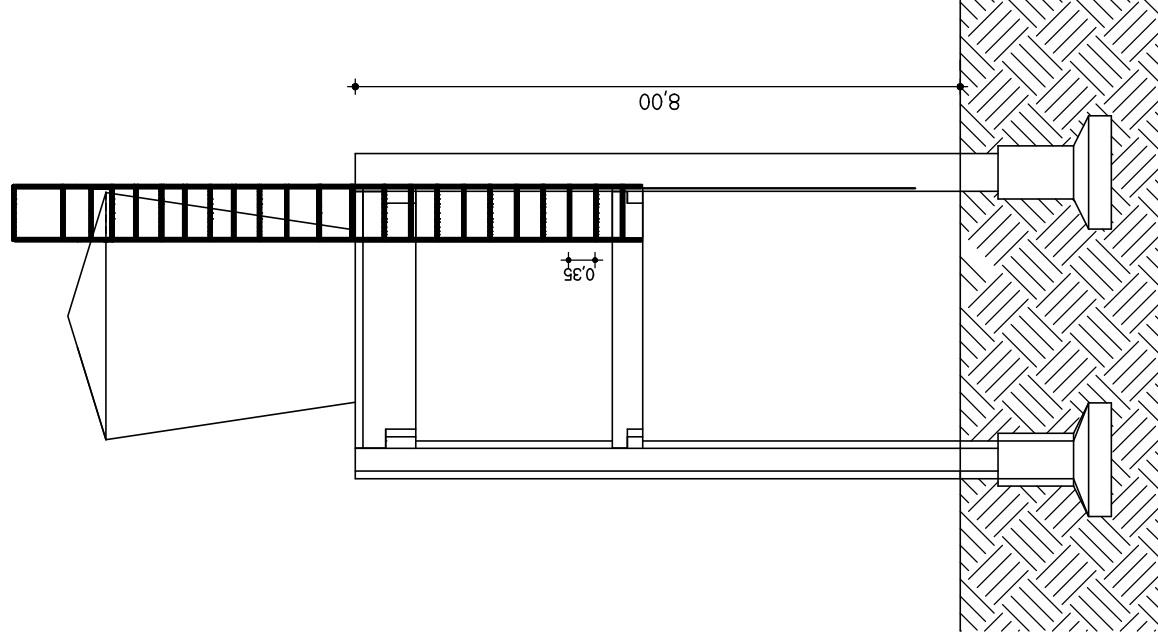
Detalhe Vertical 2 esc. 1:100
