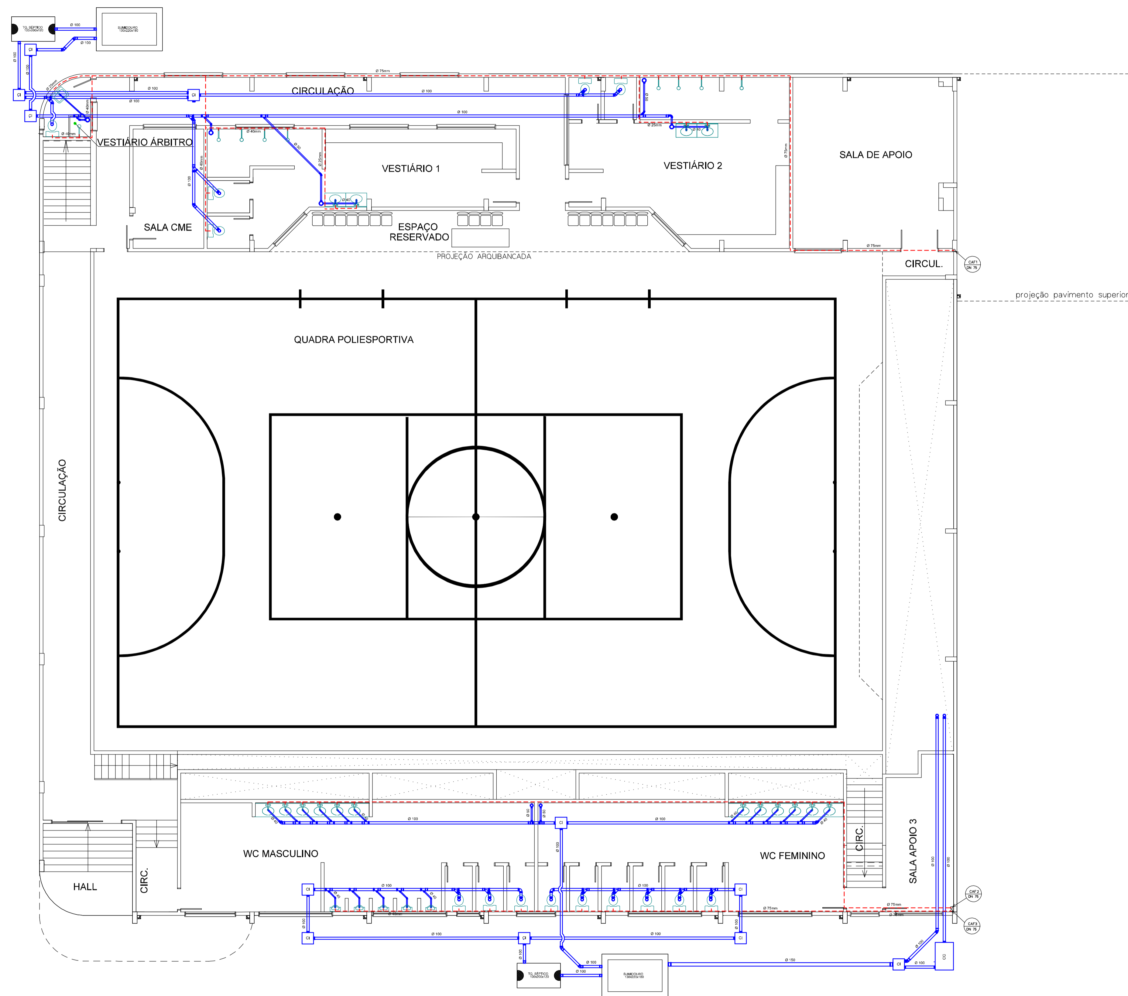
PLANTA BAIXA INFERIOR
