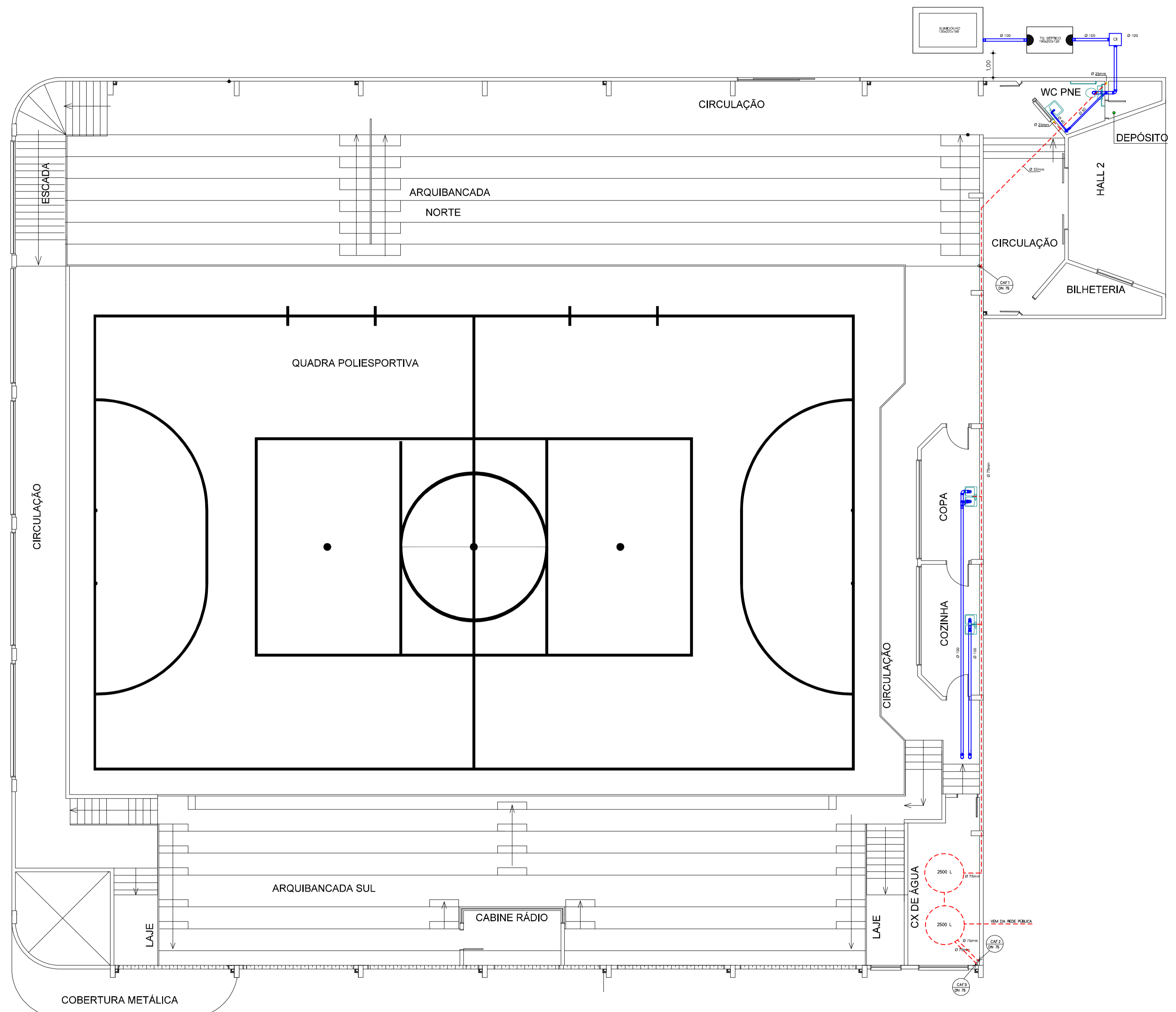
PLANTA BAIXA SUPERIOR
