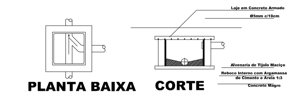
CAIXA DE INSPEÇÃO ESCALA: 1:25
