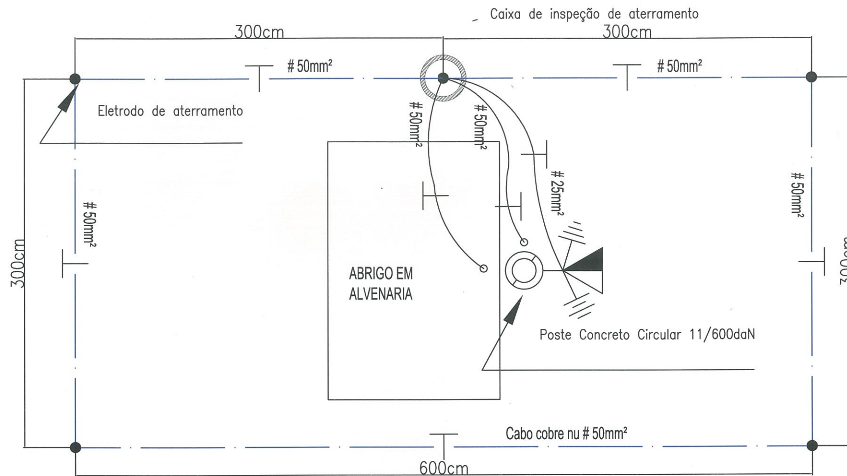
DETALHE DA MALHA DE ATERRAMENTO
